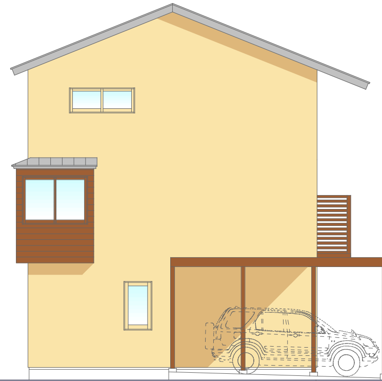
西側立面图 S: 1/100
