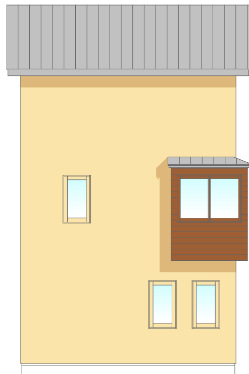
北側立面图 S: 1/100
