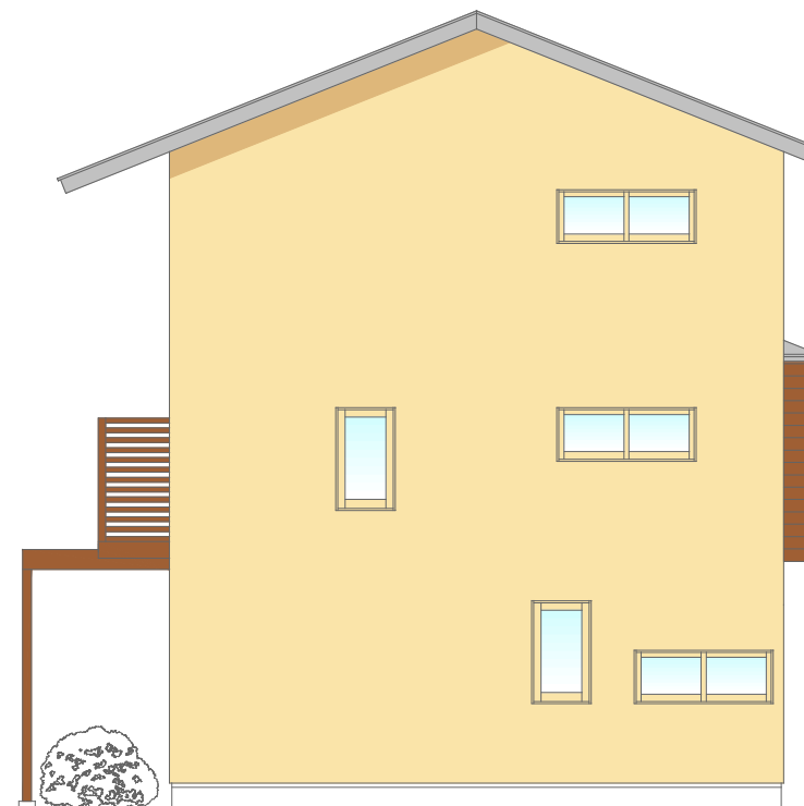
東側立面图 S: 1/100
