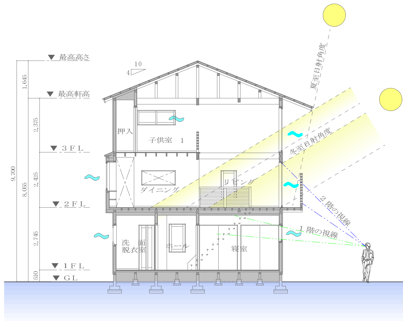
断面図 S : 1/100
