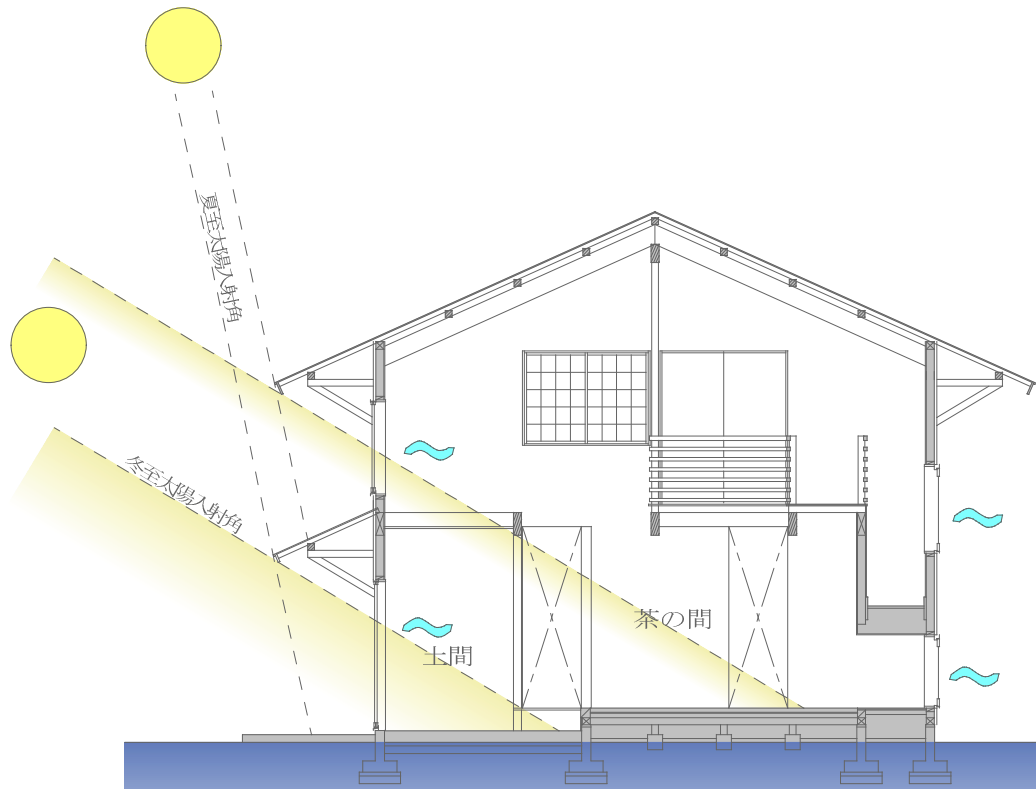
縦断面図 S: 1/100
