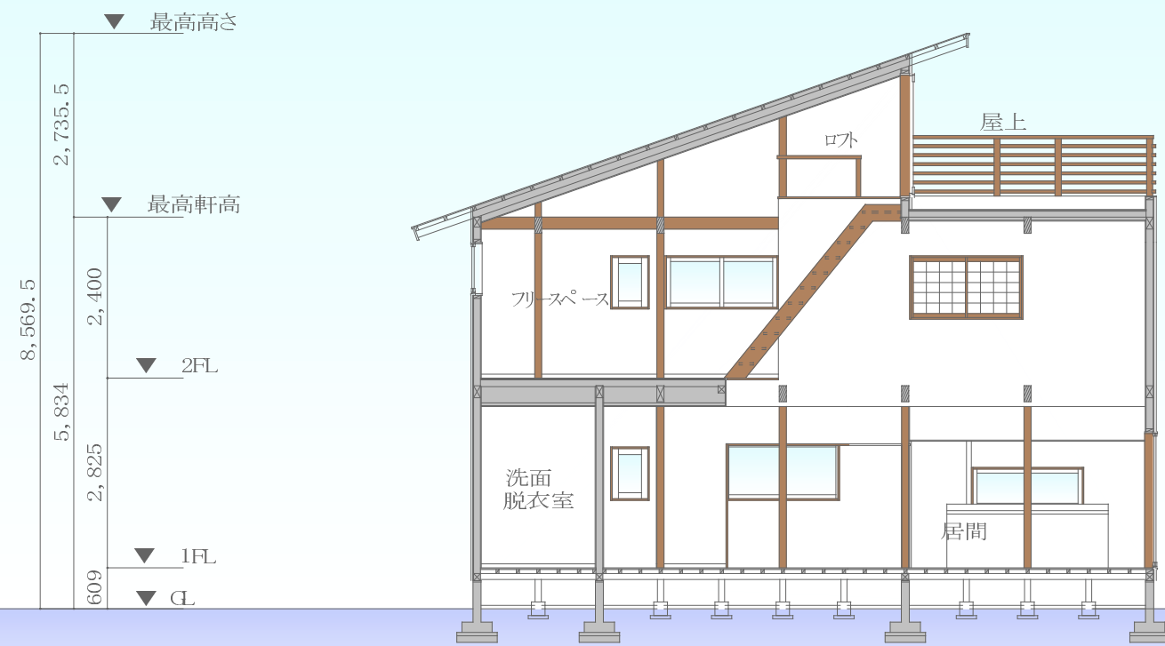
縦断面図 S: 1/100
