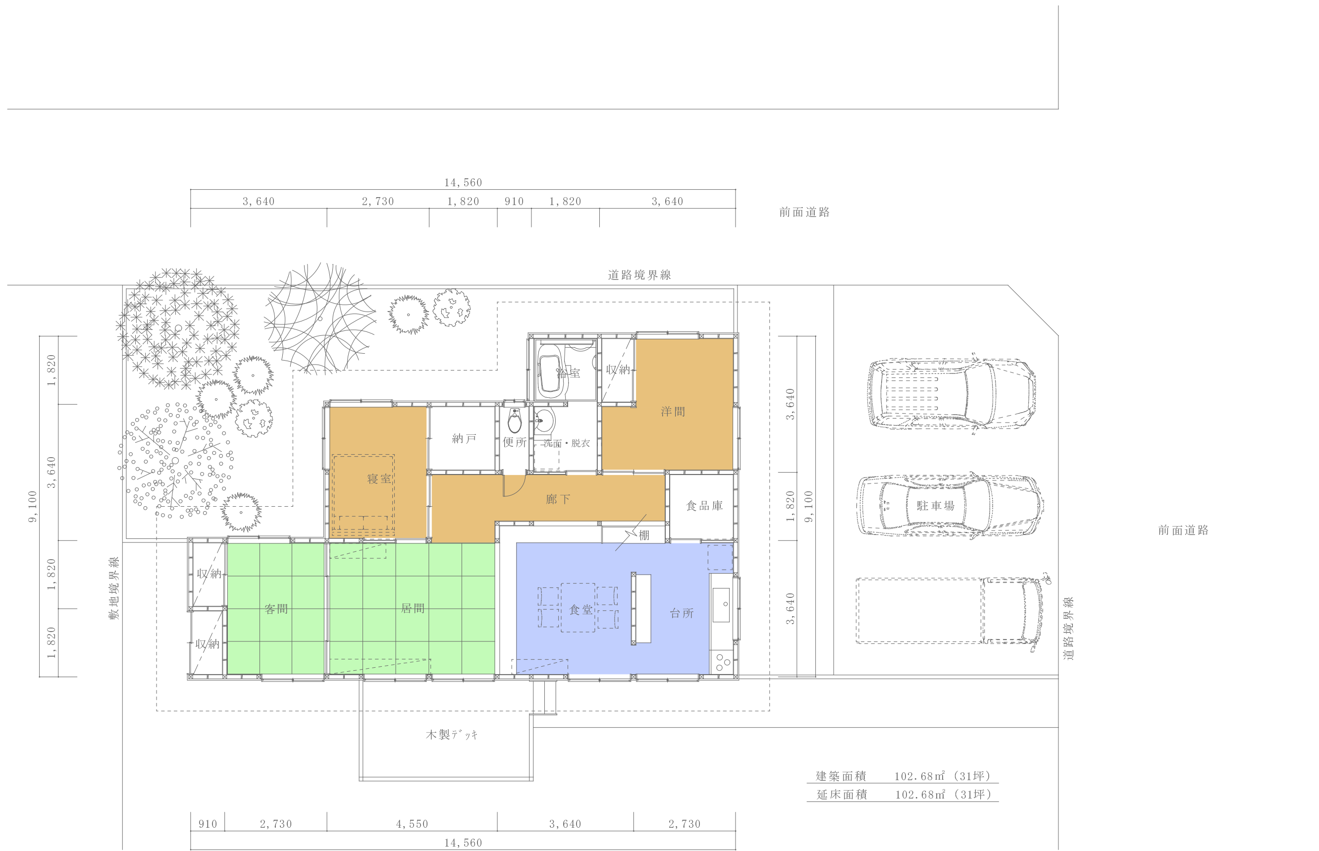
平面図 S : 1/100
